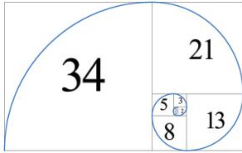
الشكل (16) مخطط النسبة الذهبية الذي صممه فيبوناتشي
