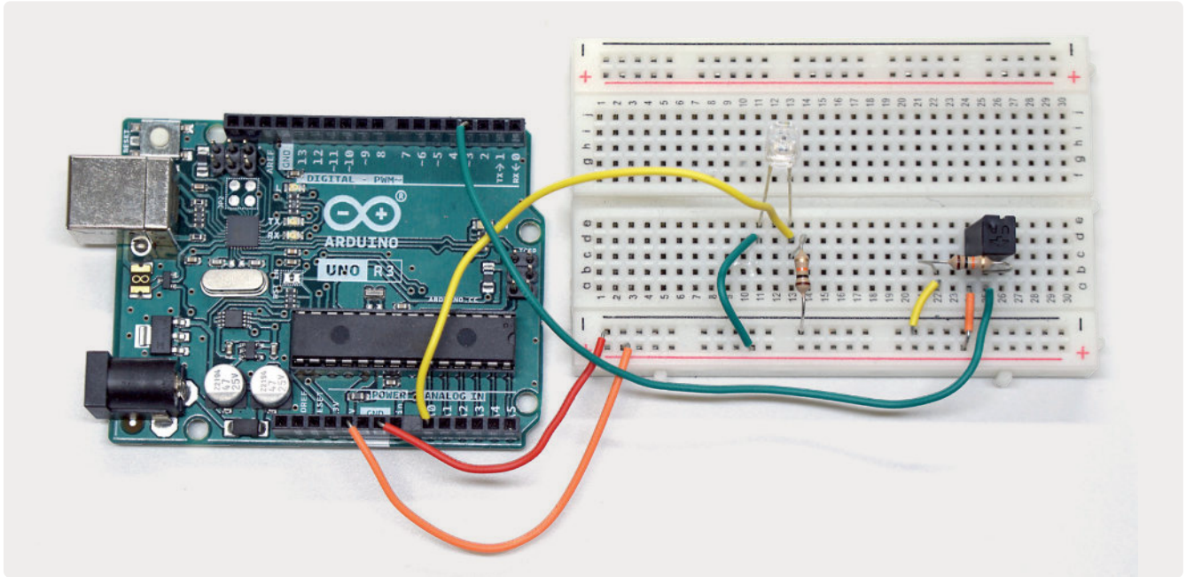
شكل 7.17: صورة للدائرة
