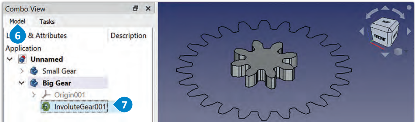
شكل 2.48: إضافة الترس الأسطواني المنحني
